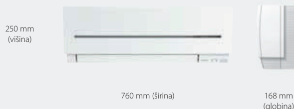
Dimenzije modelov MSZ-SF 15-20
